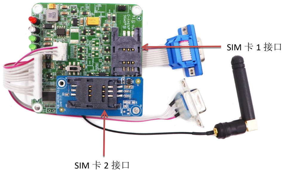
SIM/UIIM 卡安装
