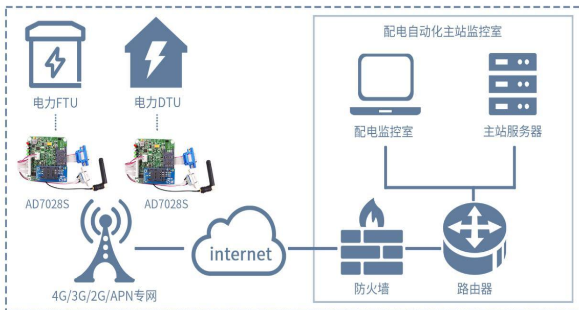
IP MODEM 应用拓扑图
